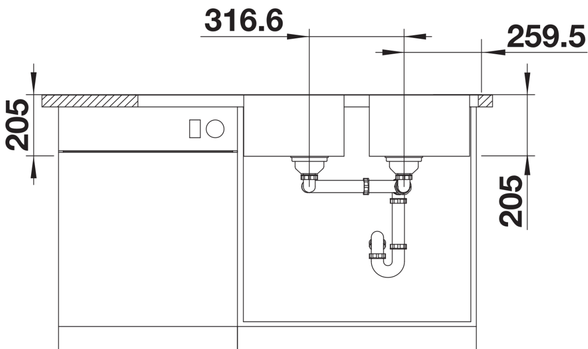
Vooraanzicht
