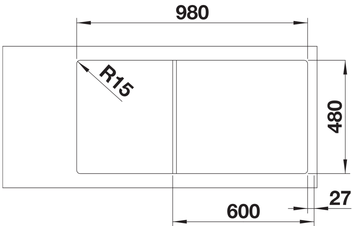
Uitgesneden
