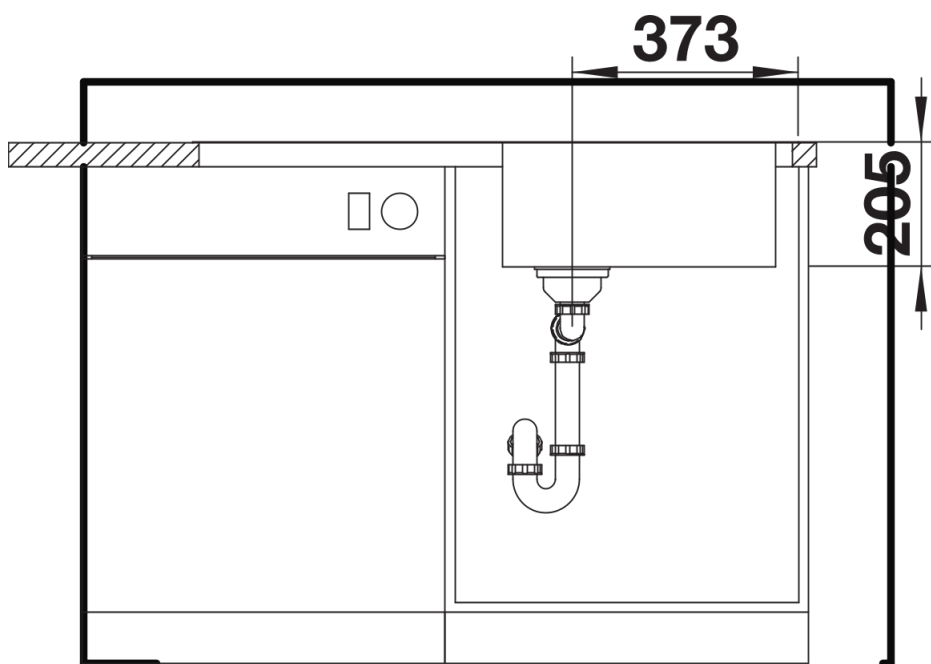
Vooraanzicht
