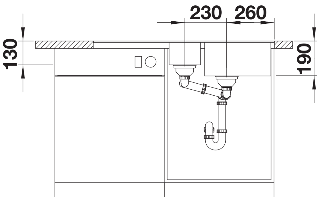
Vooraanzicht
