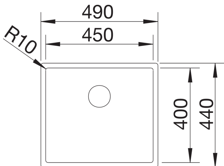
Bovenaanzicht
