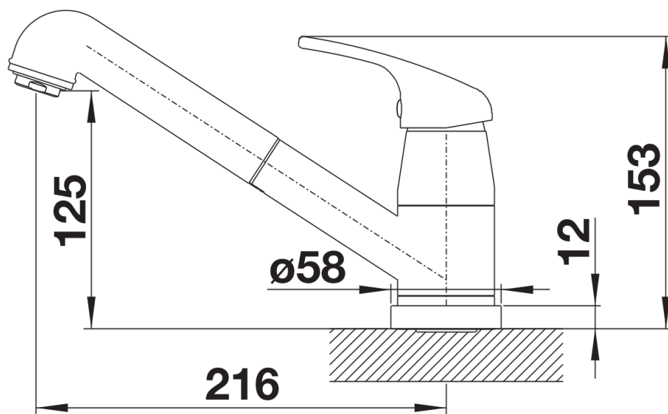
Zijaanzicht
