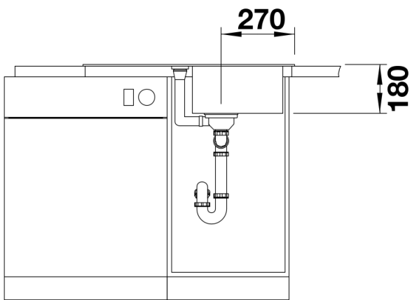
Vooraanzicht
