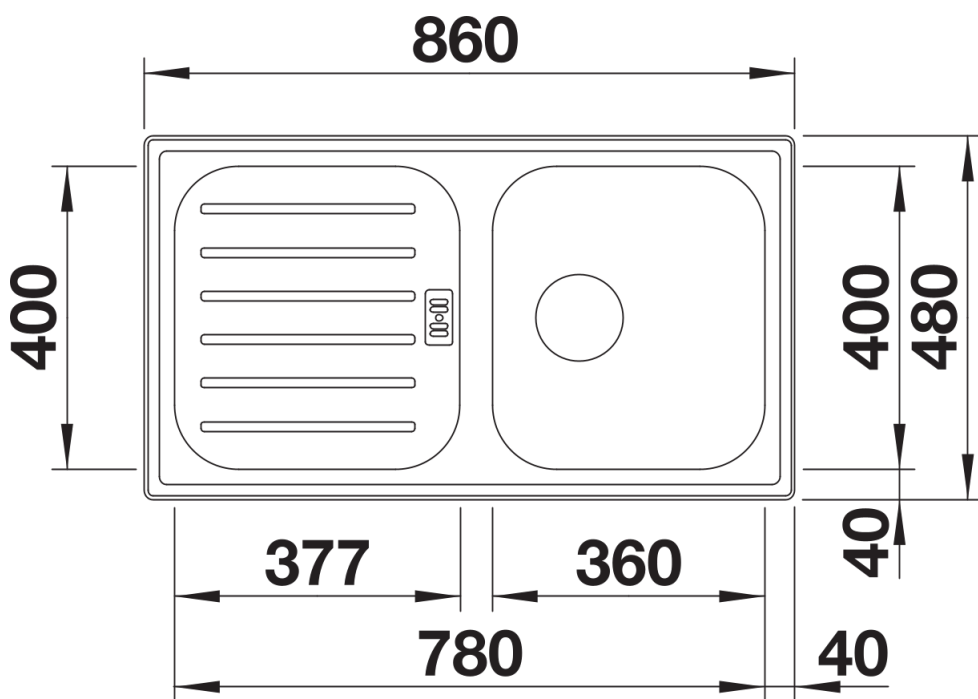
Bovenaanzicht
