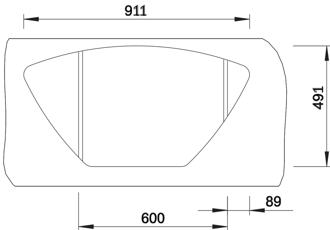
Uitgesneden
