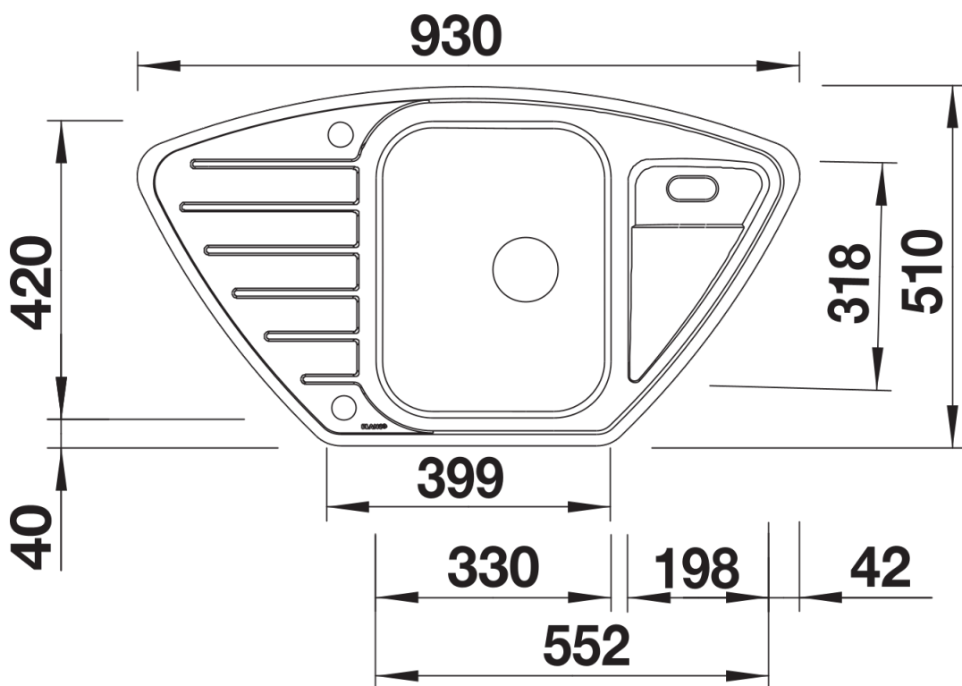
Bovenaanzicht
