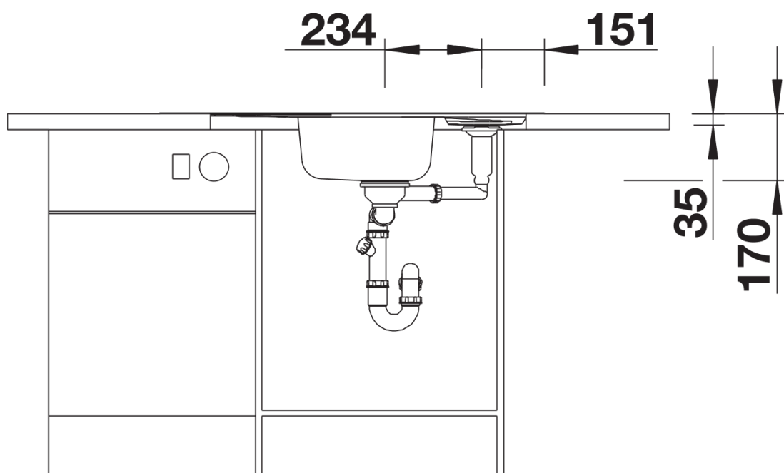
Vooraanzicht
