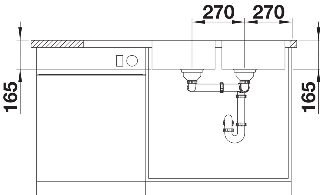
Vooraanzicht
