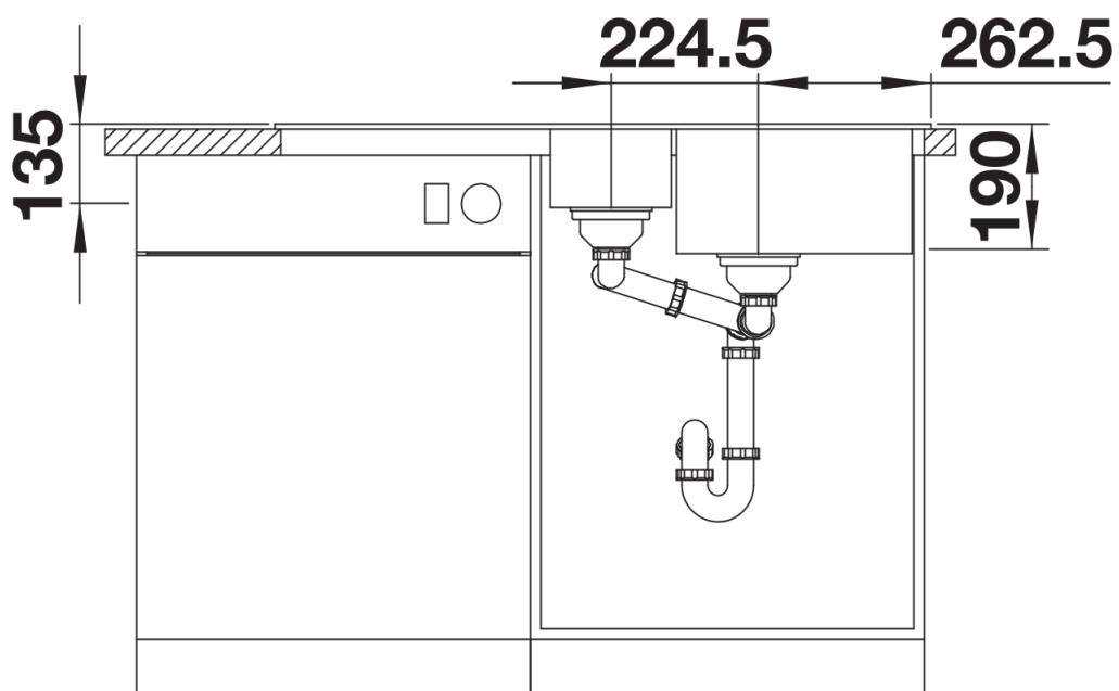
Vooraanzicht
