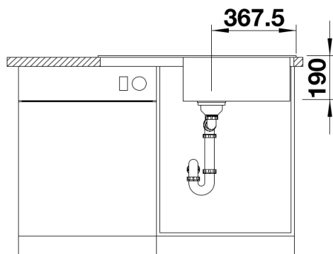
Vooranzicht
