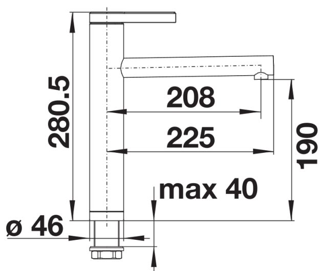
Zijaanzicht
