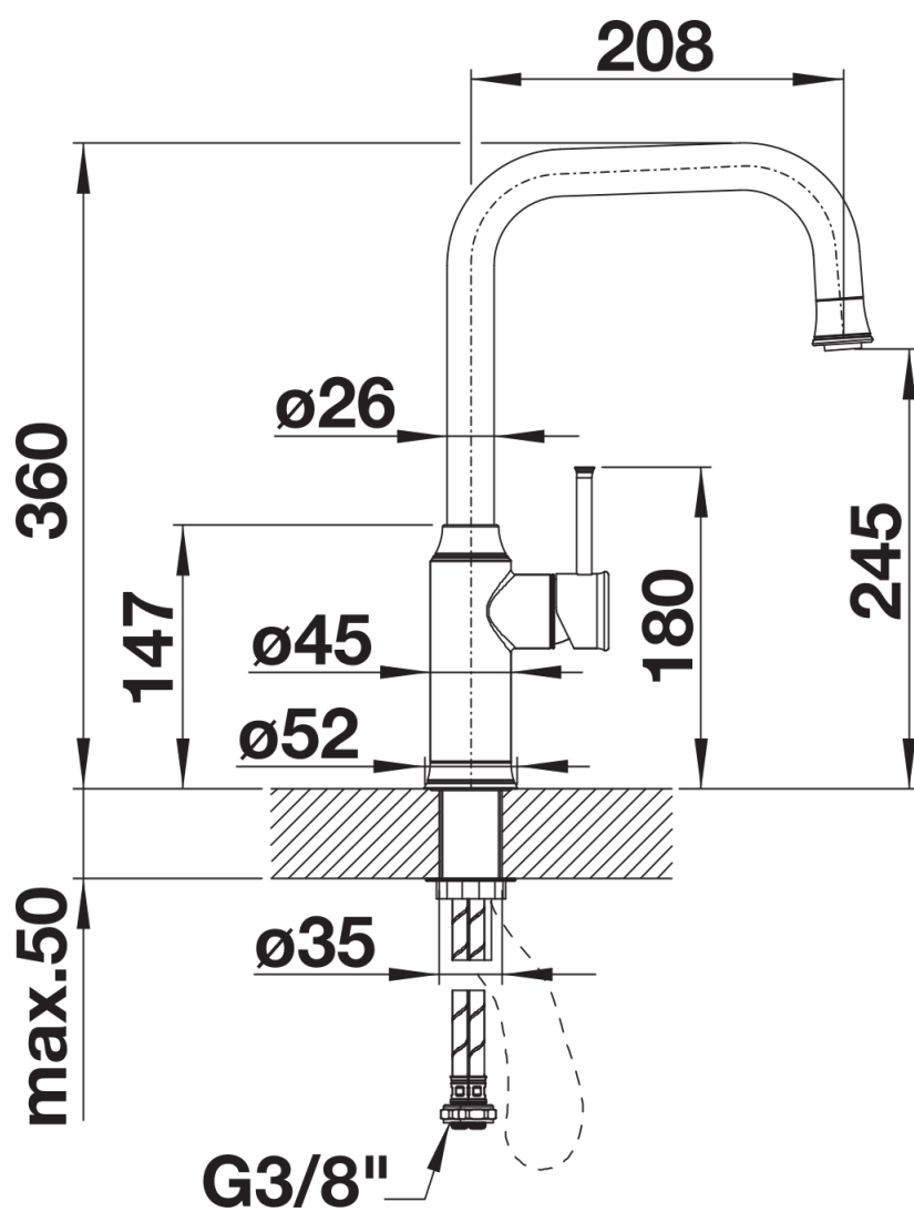
Zijaanzicht
