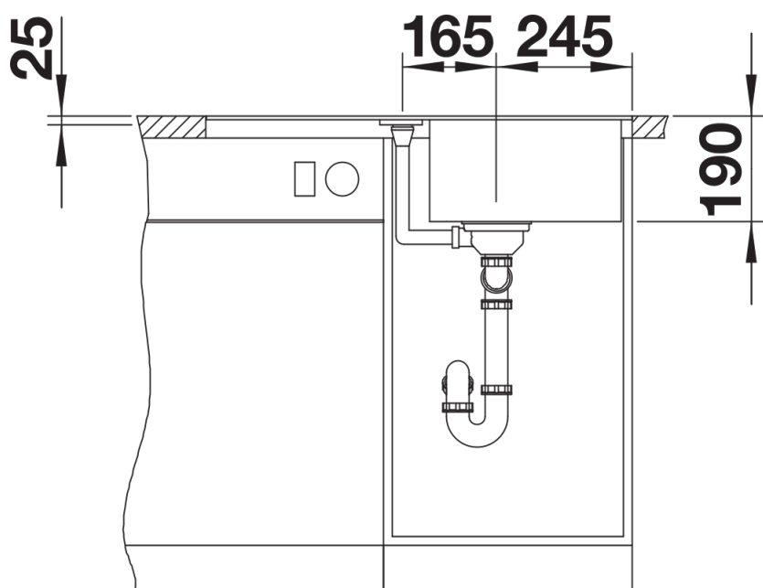
Vooraanzicht
