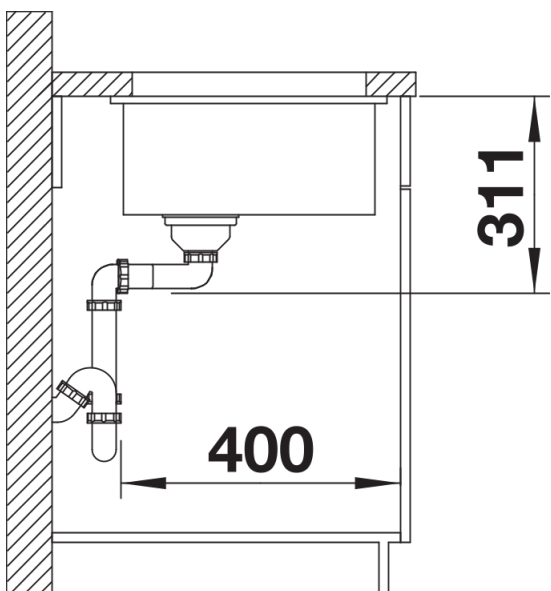
Zijaanzicht
