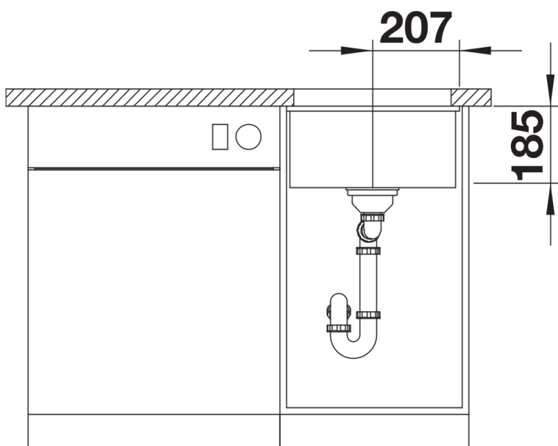
Vooraanzicht
