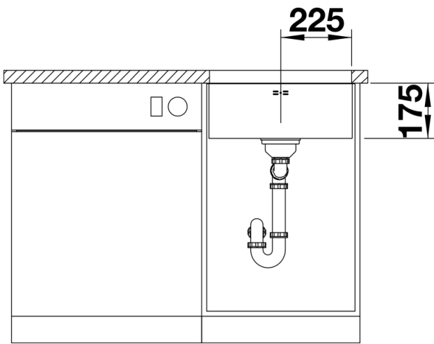
Vooranzicht
