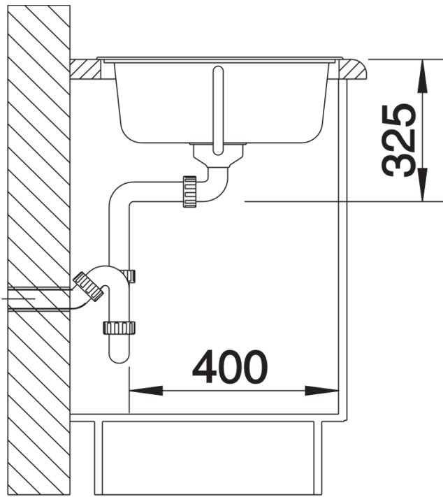
Zijaanzicht
