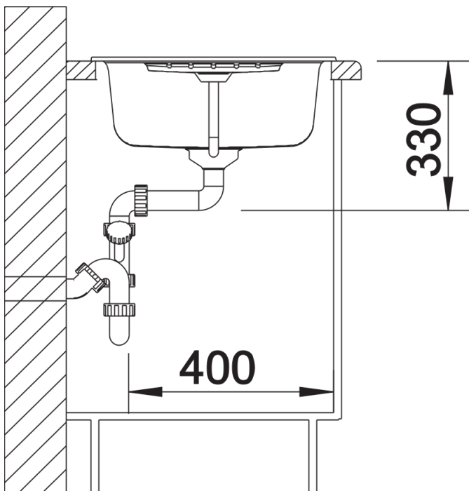
Zijaanzicht
