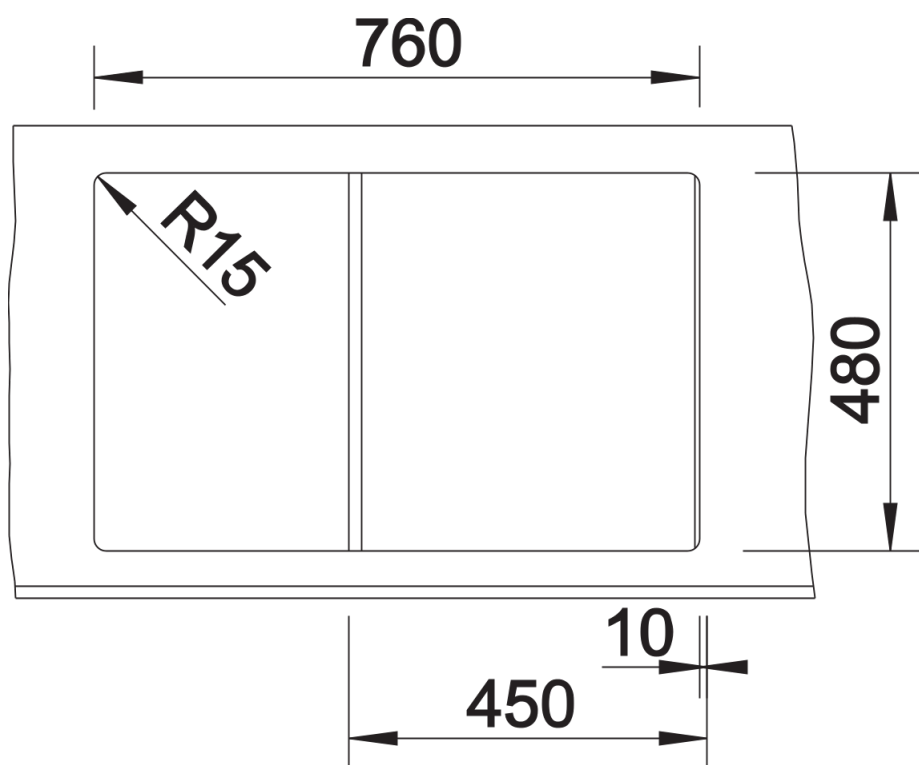
Uitgesneden
