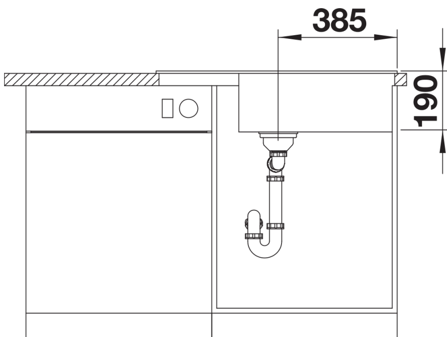
Vooraanzicht
