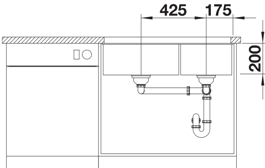
Vooraanzicht
