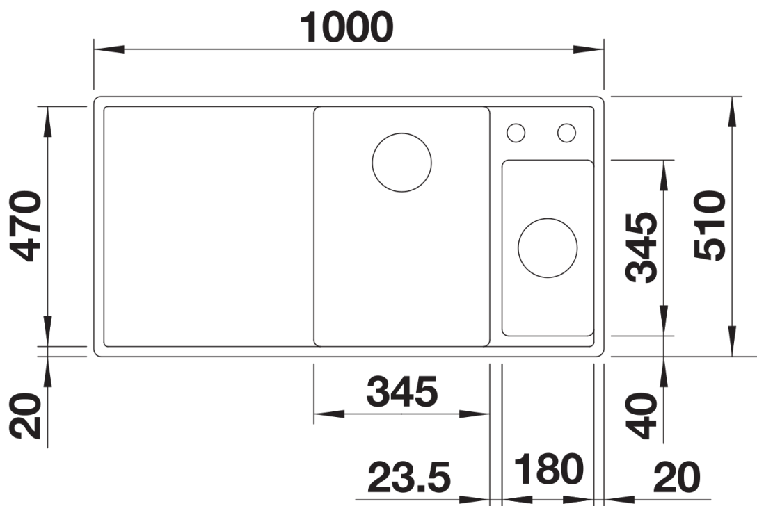
Bovenaanzicht
