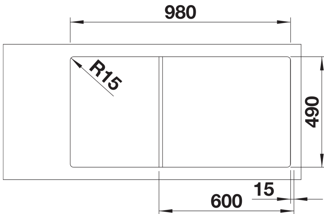
Uitgesneden
