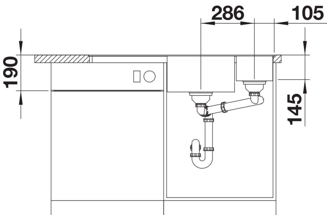
Vooraanzicht
