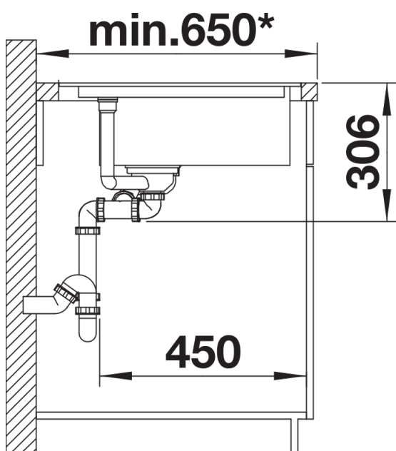
Zijaanzicht
