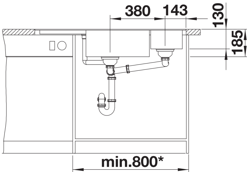
Vooraanzicht
