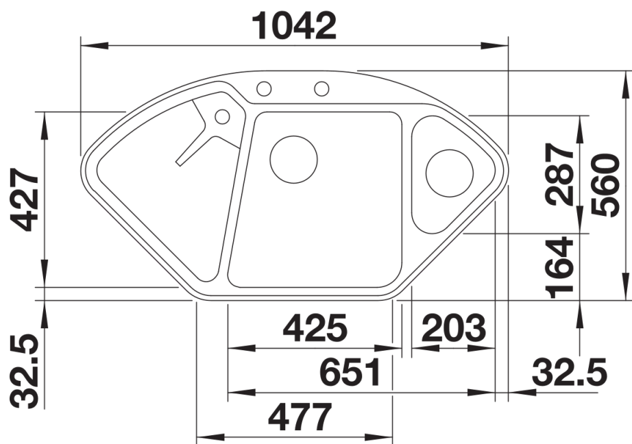
Bovenaanzicht
