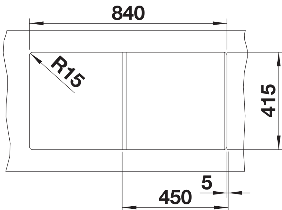
Uitgesneden
