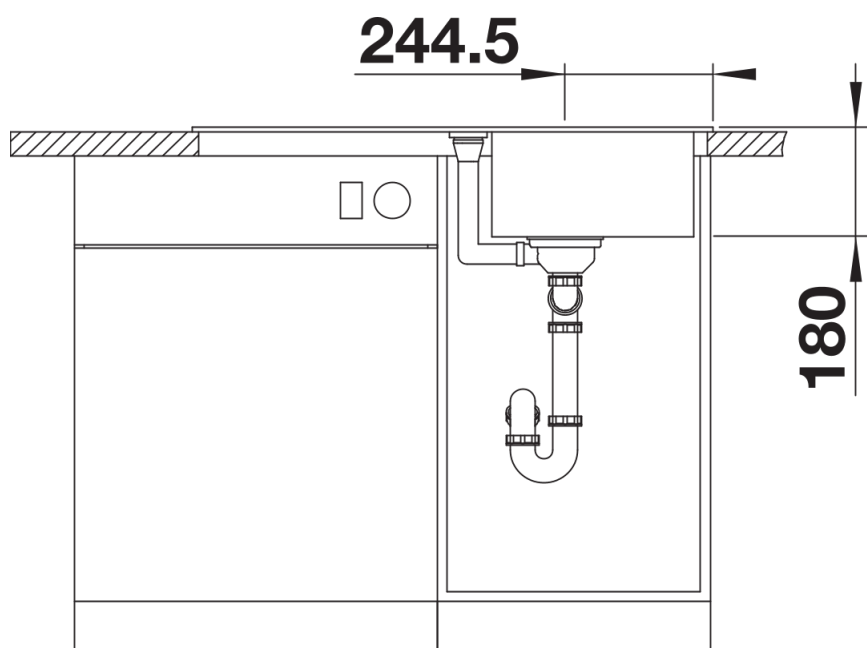
Vooraanzicht
