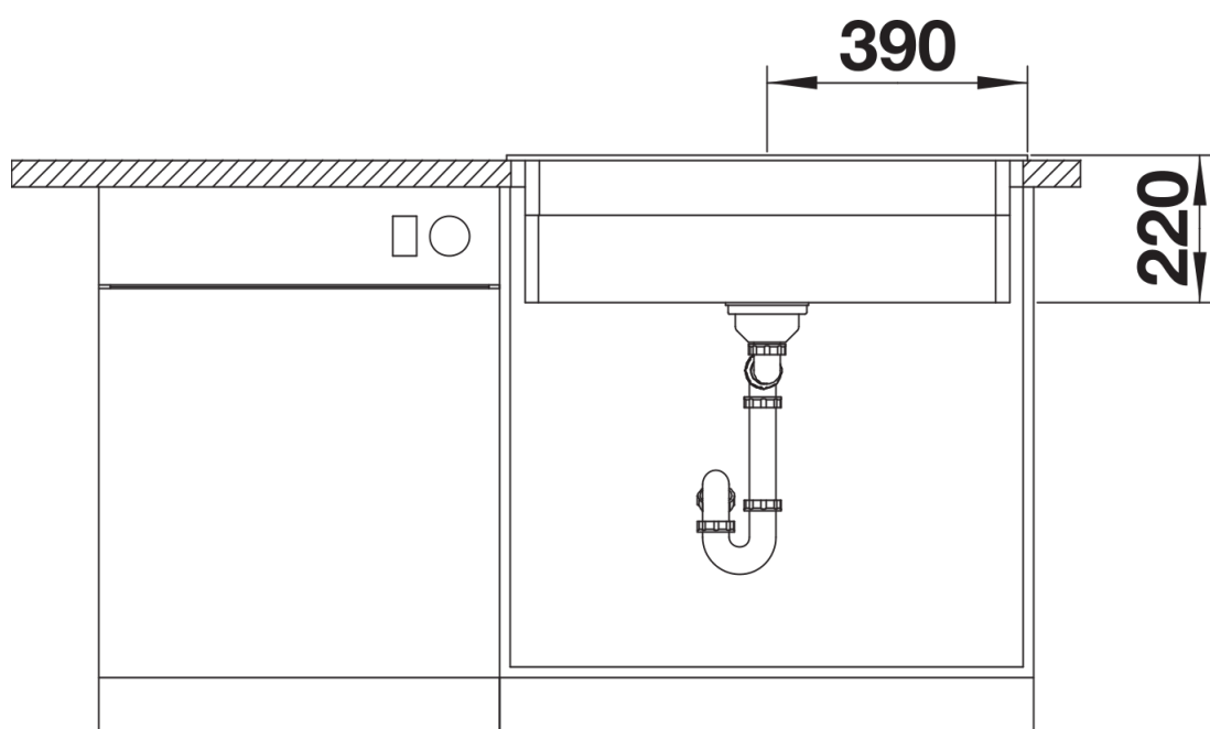
Frontansicht
