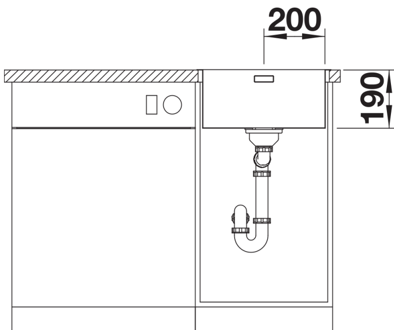
Frontansicht
