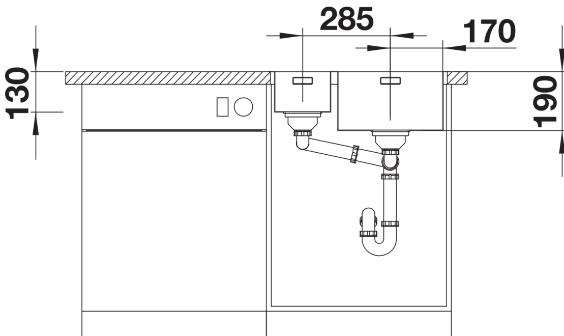
Frontansicht
