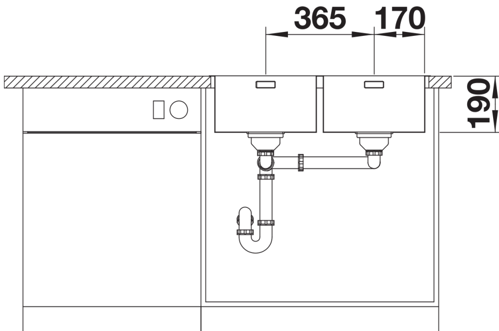
Frontansicht
