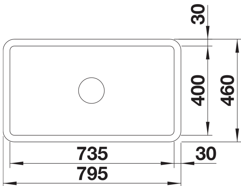
Aufsicht
