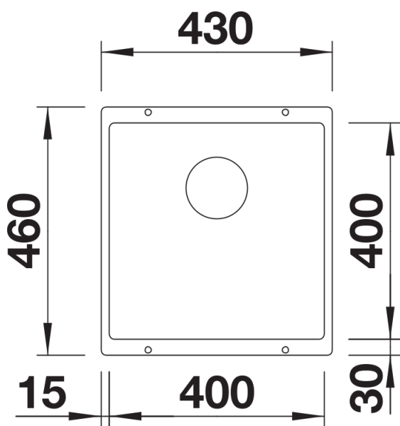
Aufsicht
