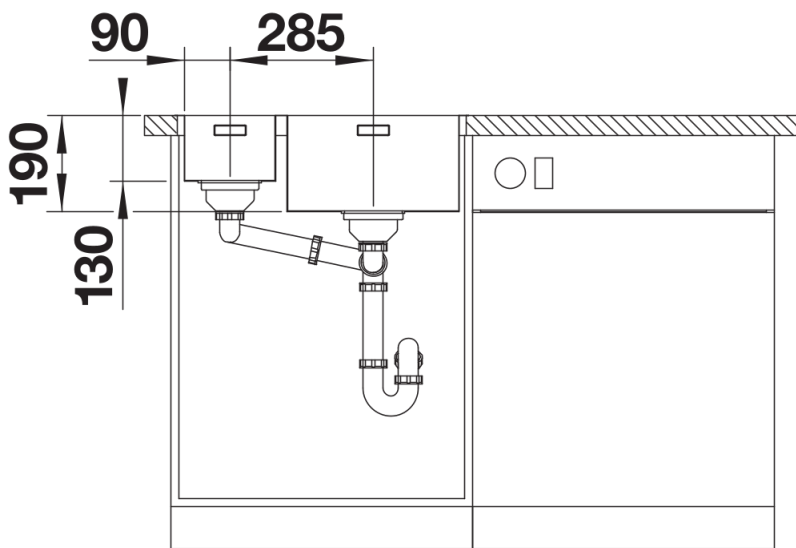
Frontansicht
