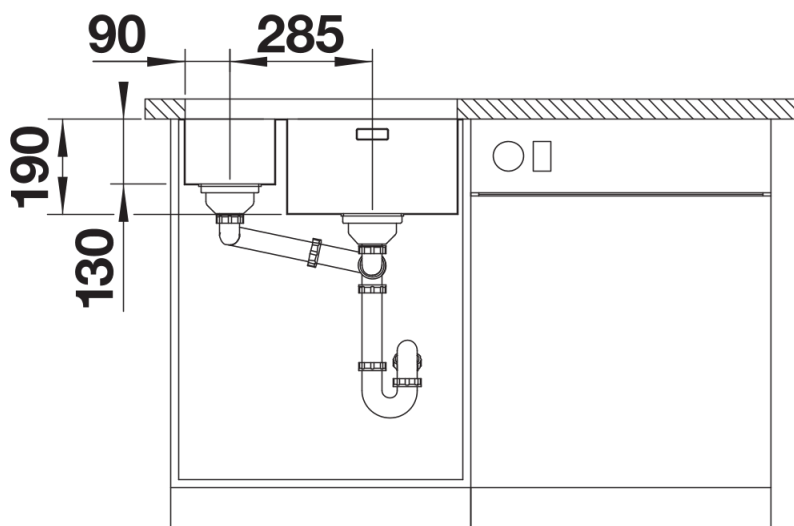
Frontansicht
