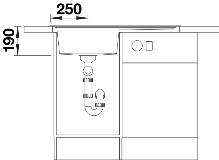
Frontansicht
