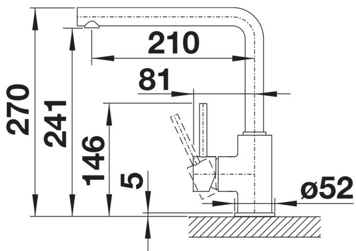
Seitenansicht
