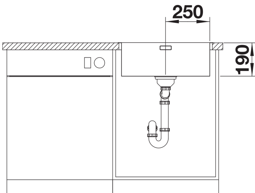
Frontansicht
