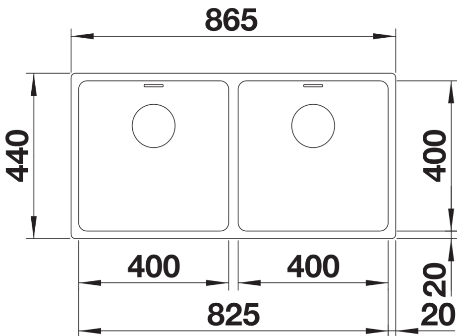
Aufsicht
