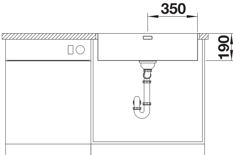
Frontansicht
