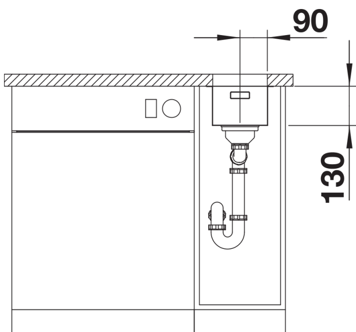
Frontansicht
