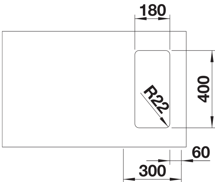
Ausschnitt
