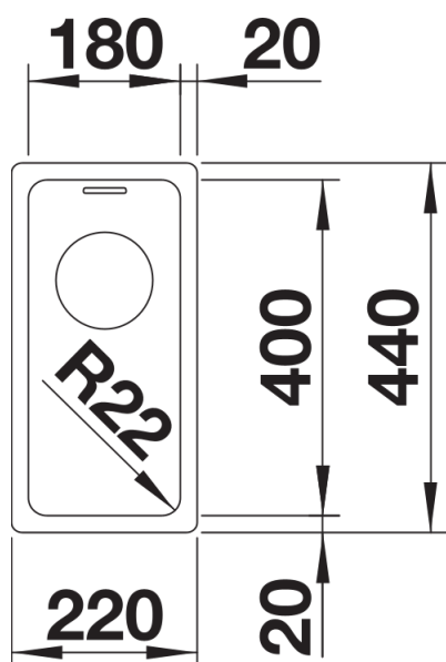
Aufsicht
