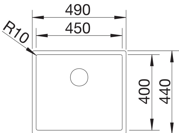
Aufsicht
