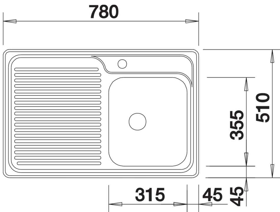
Aufsicht
