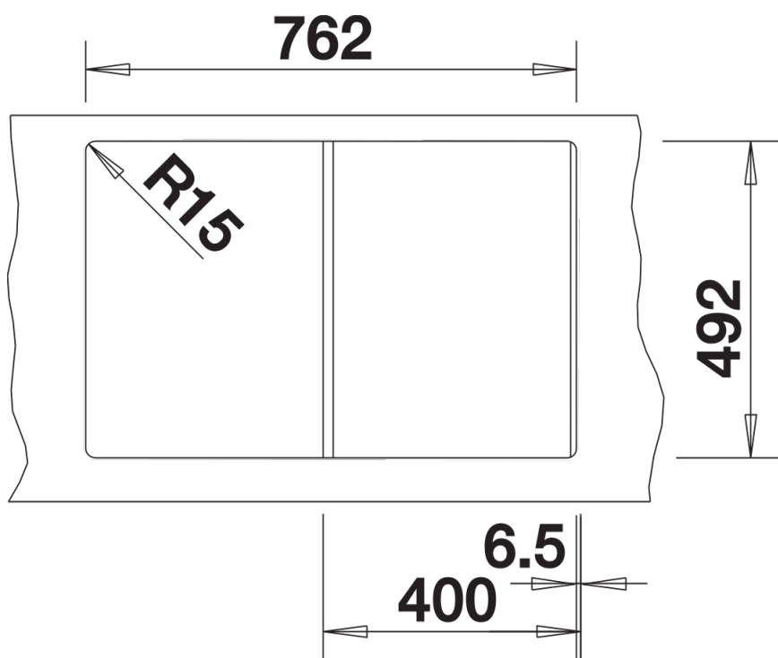
Ausschnitt
