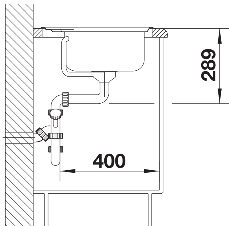
Seitenansicht
