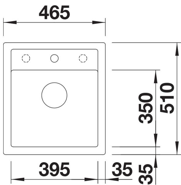
Aufsicht
