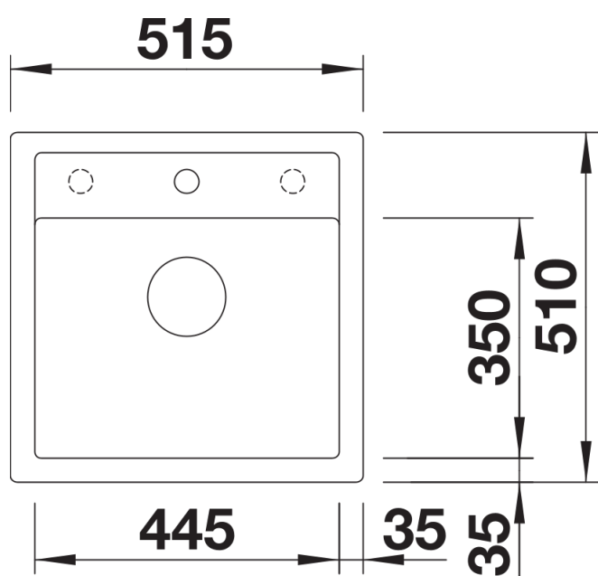
Aufsicht
