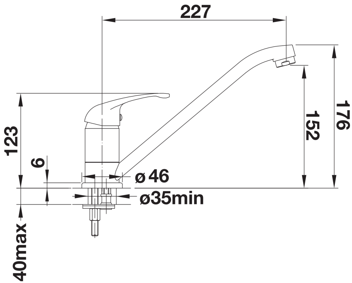
Seitenansicht
