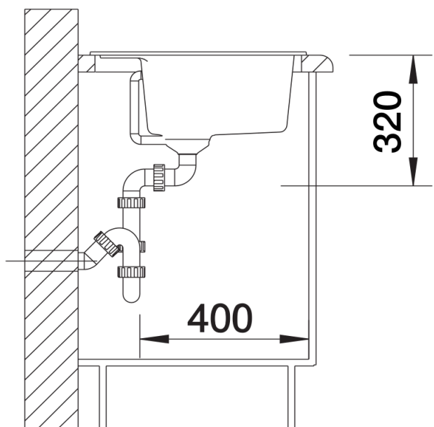
Seitenansicht
