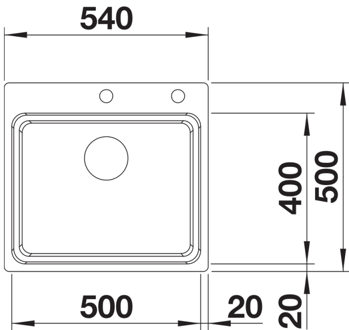
Aufsicht
