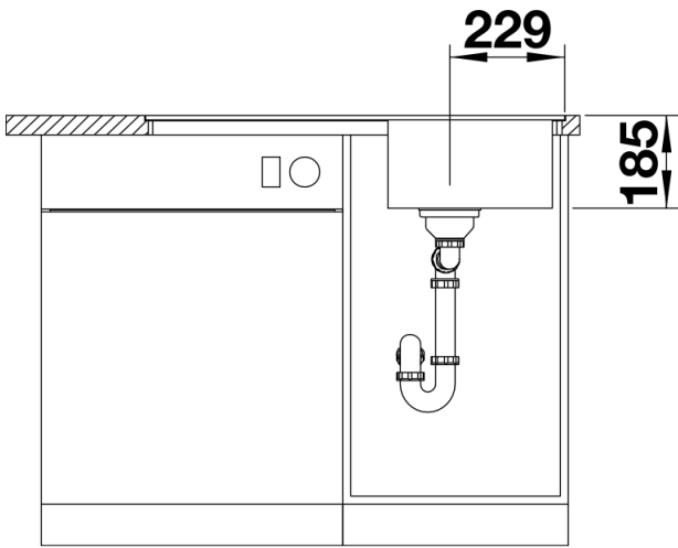
Frontansicht
