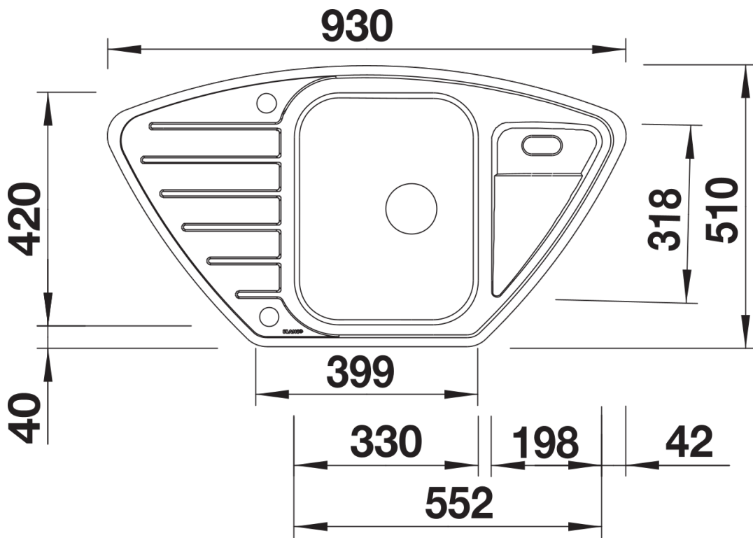
Aufsicht
