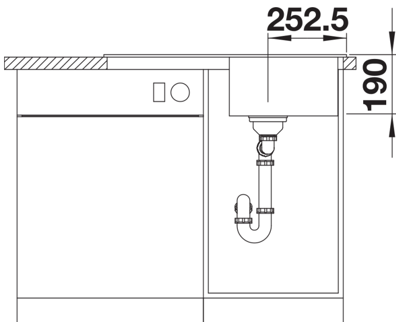
Frontansicht
