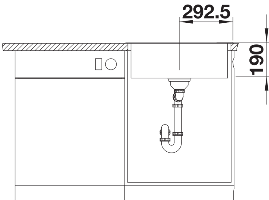
Frontansicht
