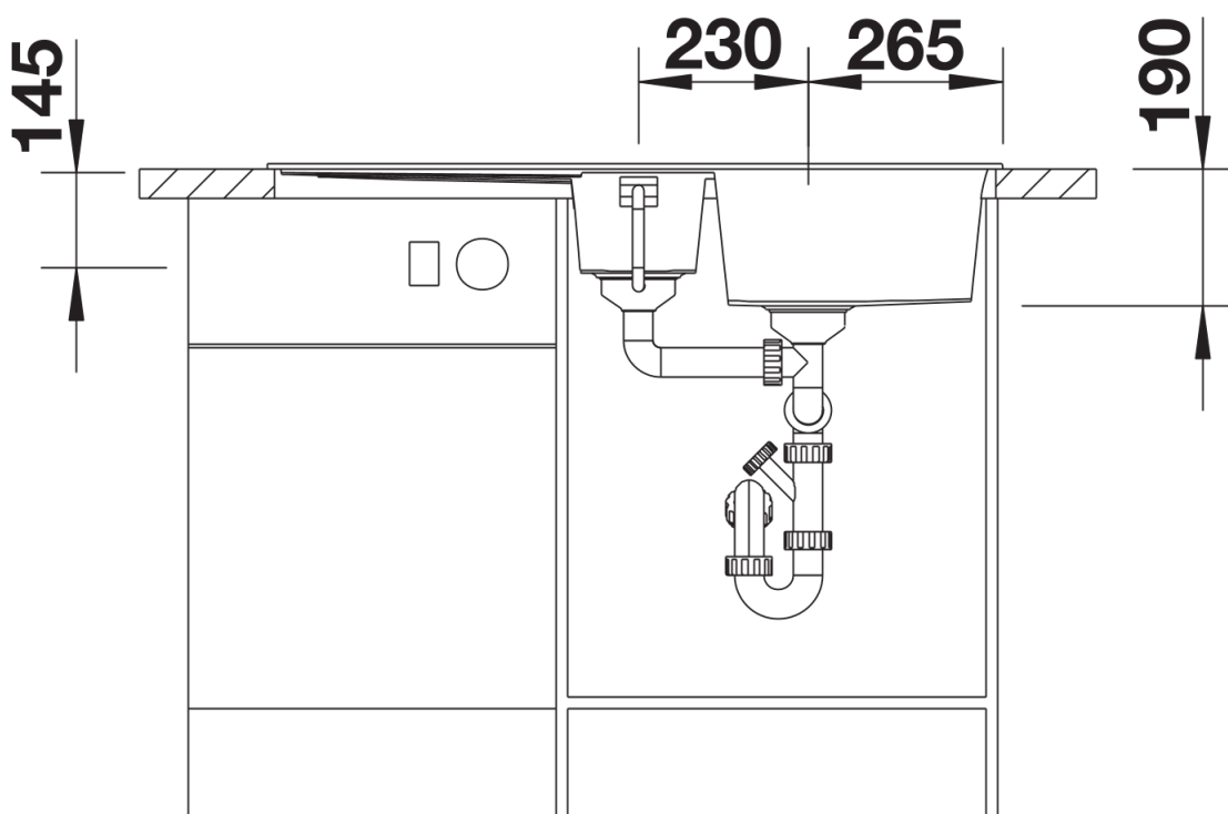
Frontansicht
